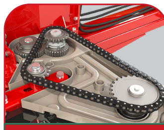
Transmisión por cadena
