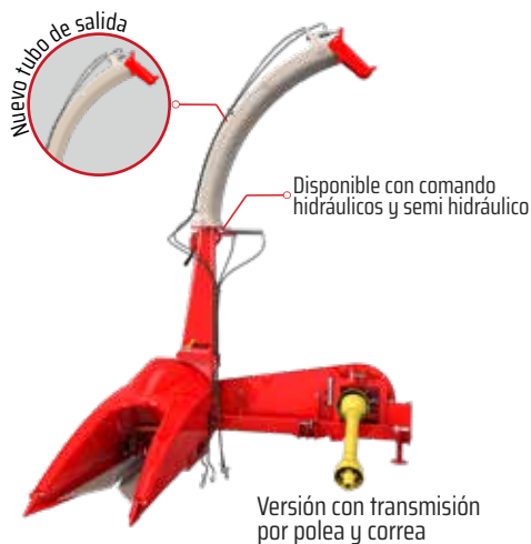
Articulación sencilla para mantenimiento
